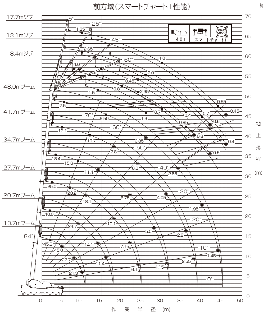
スマートチャート1性能の範囲 (アウトリガ最大張出時)
